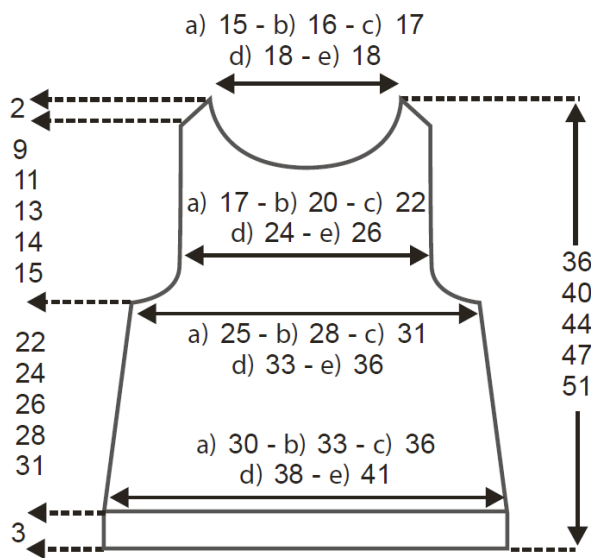
Skabelon til forstykke
